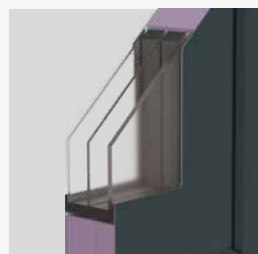
TRIPLE VITRAGE Feuilleté 33.2 retardateur d'effraction
